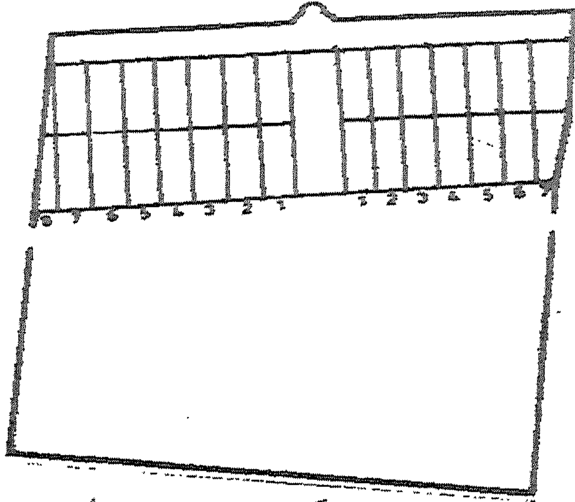
(شكل رقم ٦٧) رسم افتراضى لمخطط جامع الزيتونة فى حالة وضح الأروقة متعامدة تماما مع جدار القبلة عن د/الدولاتلى .
